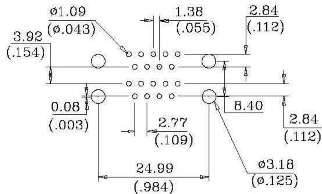
P.C.B LAYOUT
